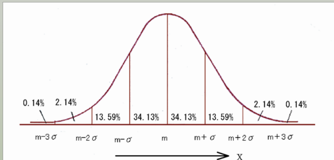
正規分布
